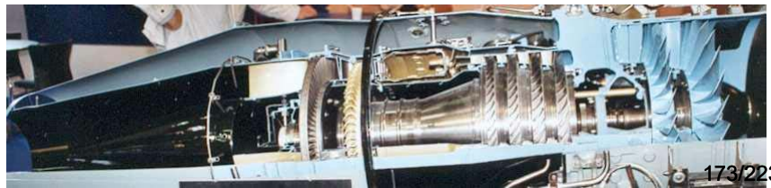
Réacteurs double corps – double flux : civil de chez PW et militaire (LARZAC – a jet).
